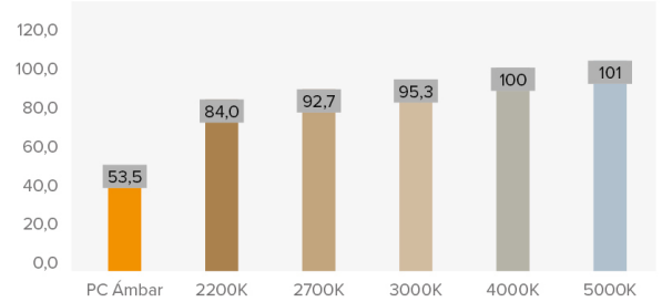
Relación Eficiencia (%) lm/W - Temperatura de Color (K)
