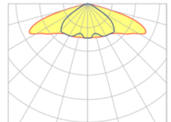
Simétrico Extensivo (SE)
