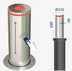
TELESCÓPICA AUTOMÁTICA Ø220 x 600mm H6008
